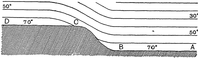
चित्र ३६ : पठार तथा मैदान पर समतापीय सतहें
